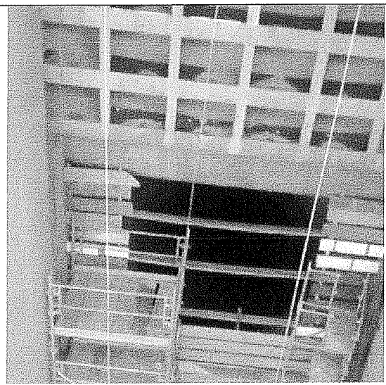
Comporta da Unidade 3 – Peso: 20 Ton
